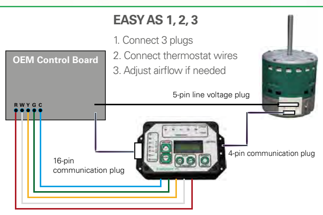
Genteq ECM model 2.3 motor
